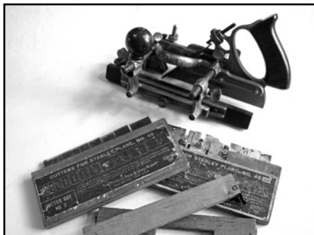
26. Stanley 45, compleet met alle beitels en onderdelen in fraaie kist. De beitetkistjes zijn origineel.
