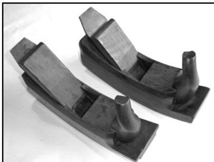
6. Set houten toogschaven, waarvan één een sponningschaaf. Fruitbomenhout, in prachtige staat.
