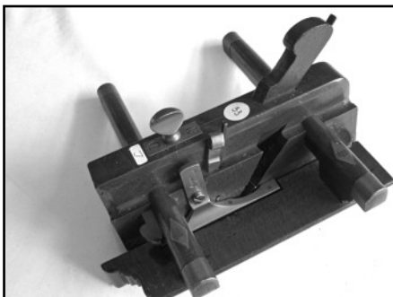
33. Engelse raamspinningschaaf van Hill. Inleg van palmhout met prachtige zwaluwstaart. Veel messing.
