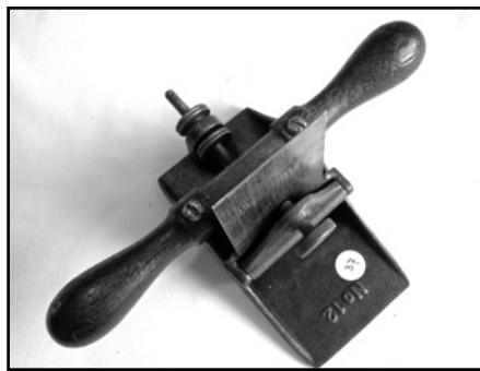
37. Stanley 12. Eerste type van omstreeks 1860-1870. IJzer niet origineel.
